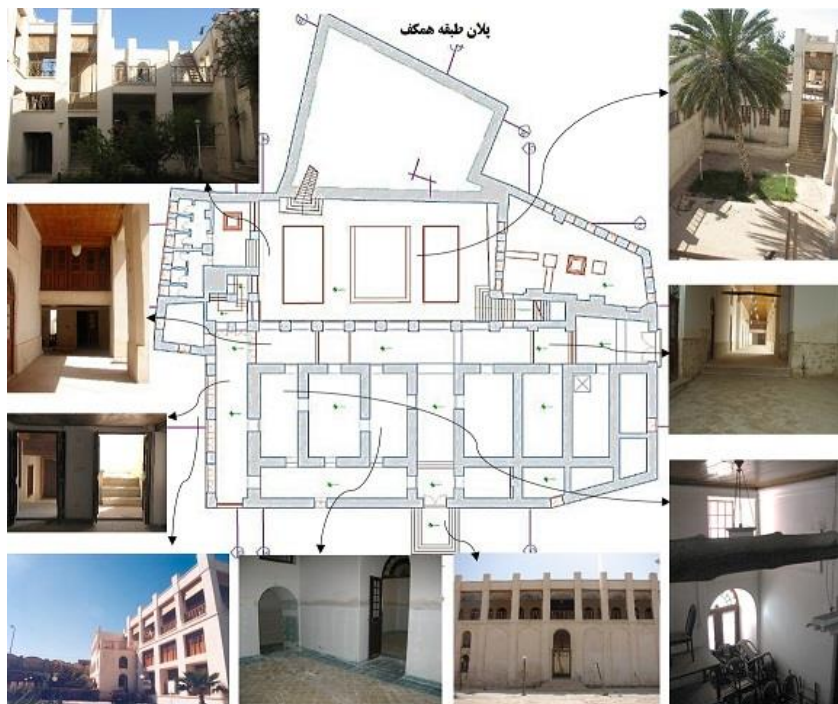
تصویر ۷. پلان طبقه همکف خانه کازرونی، منبع نگارندگان
